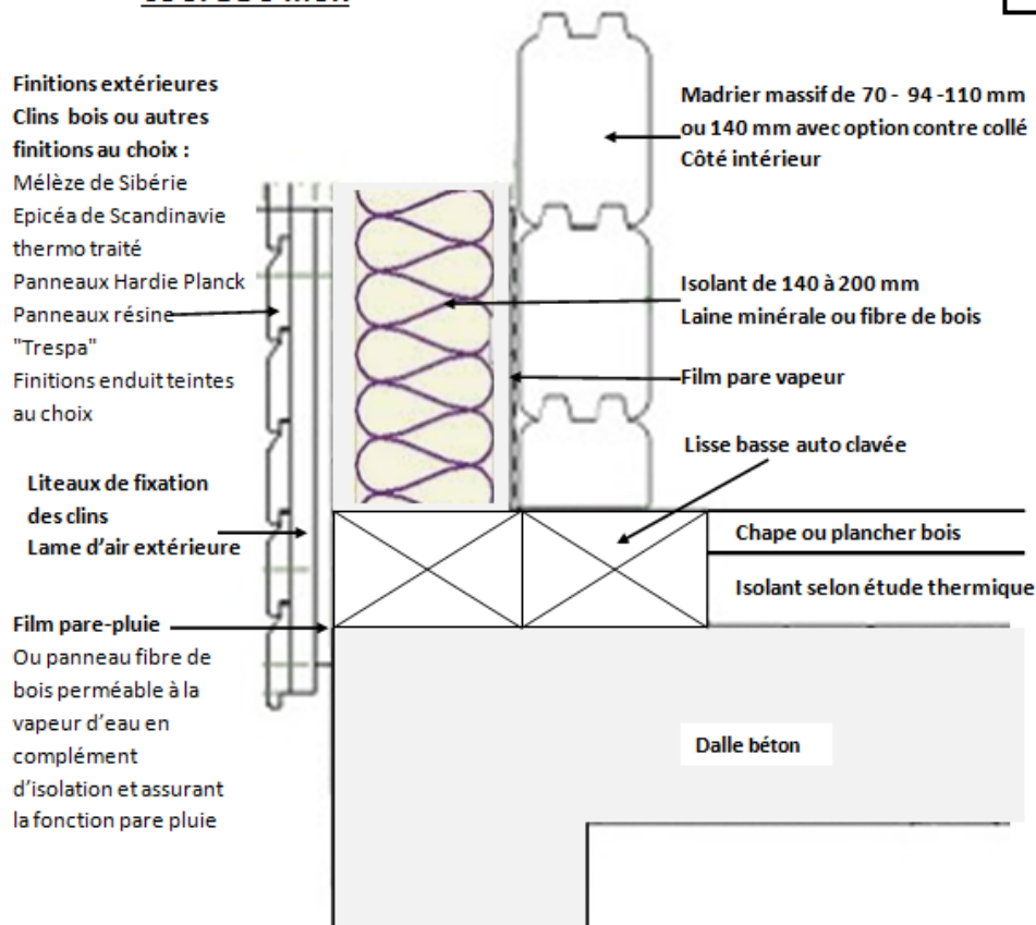
COUPE DU MUR
